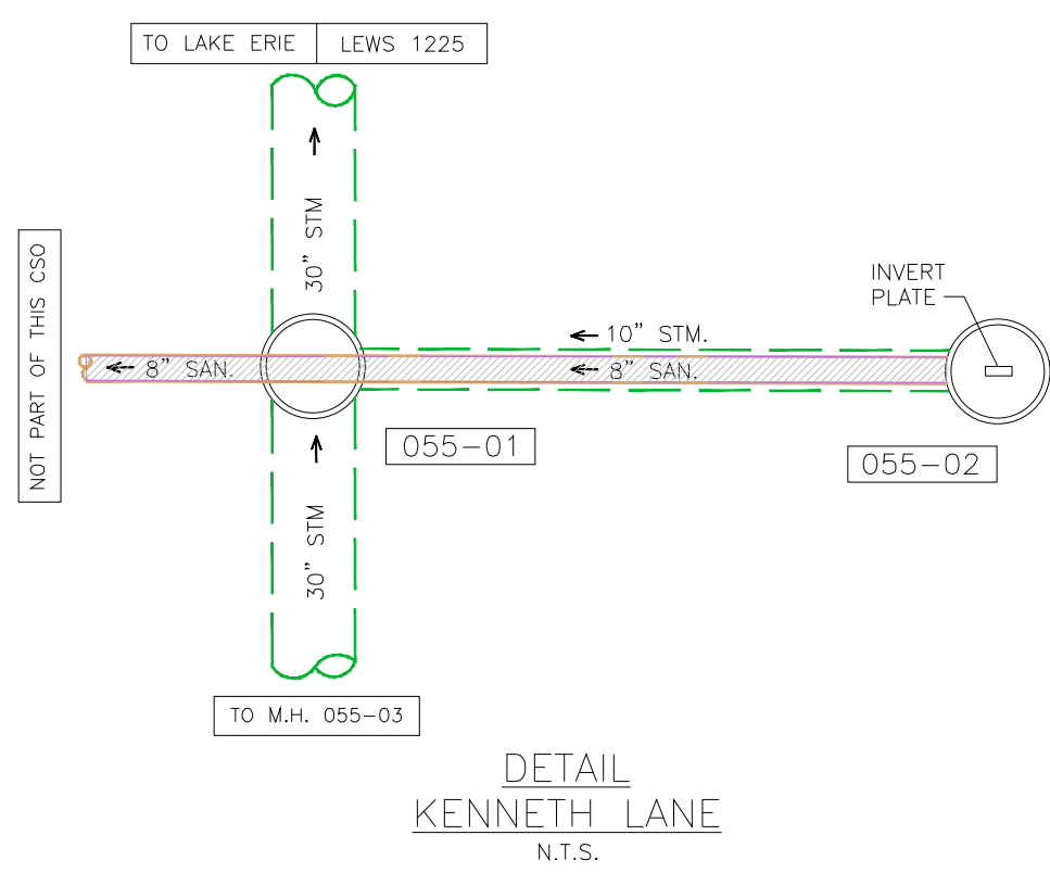
OVERFLOW 055 LEWS-1225 N.T.S.
