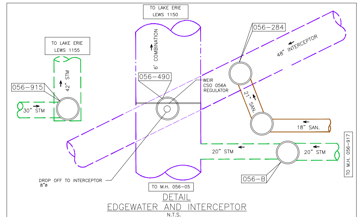
OVERFLOW CSO-056 LEWS-1150 & LEWS 1155 N.T.S.
