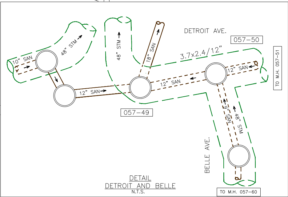
DETAIL DETROIT AND BELLE N.T.S.
