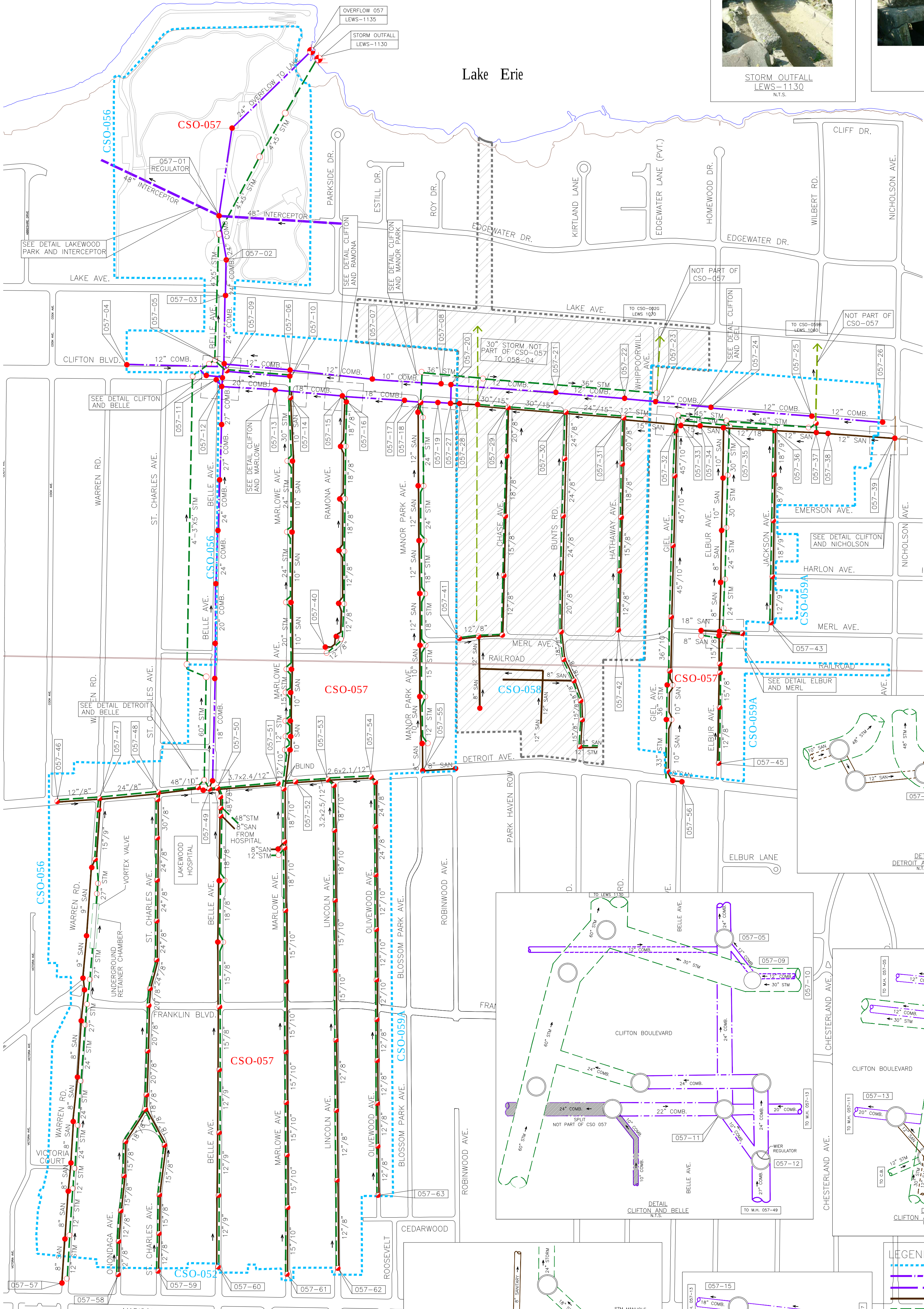
OVERFLOW 057 LEWS-1135 N.T.S.
